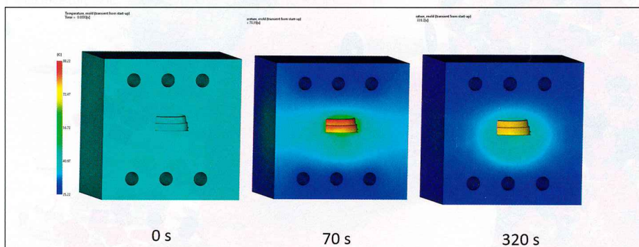
Vývoj teploty formy od začátku výroby
